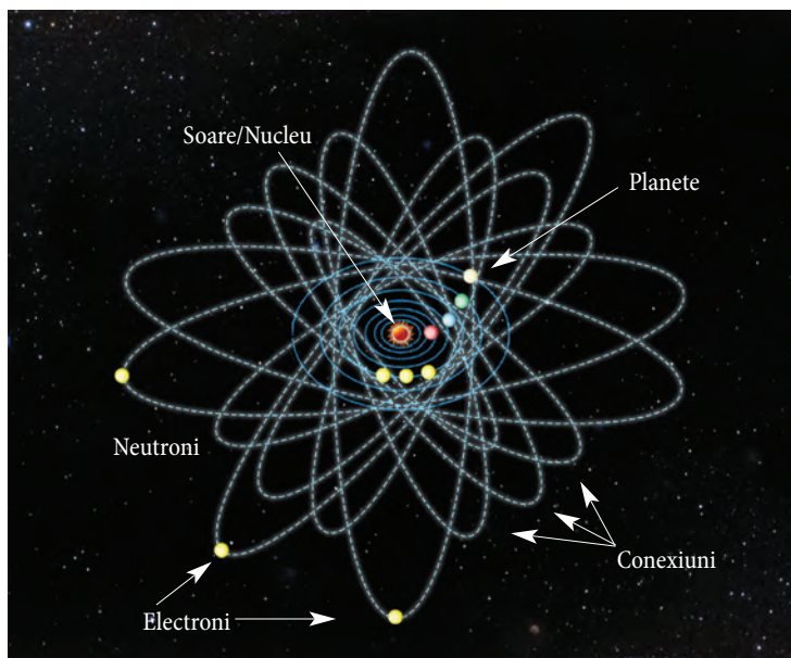
Fig. 1.7. Atomul și planetele
