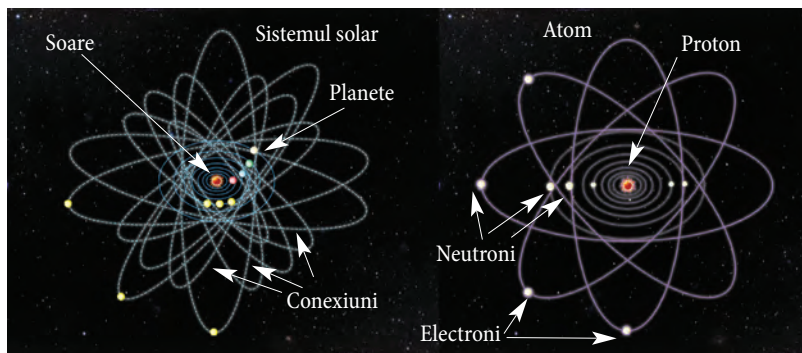
Fig. 1.6. Structura atomică și structura sistemului solar sunt asemănătoare.
